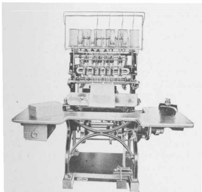
Sitomo-ompelukone.
